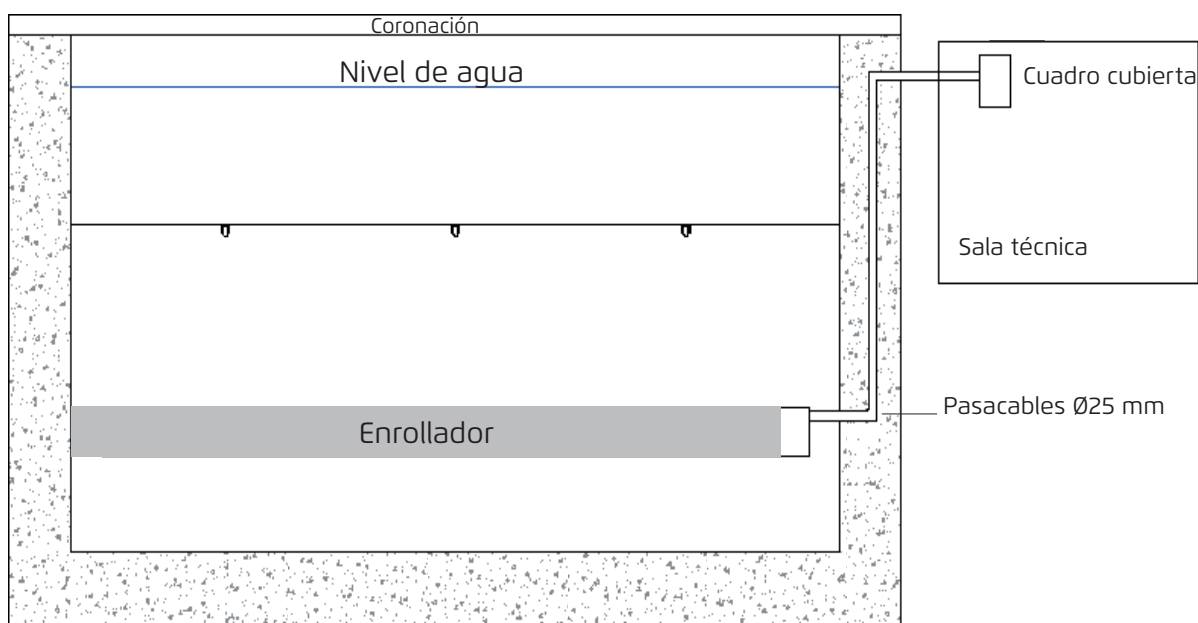
VISTA FRONTAL DEL CAJÓN
